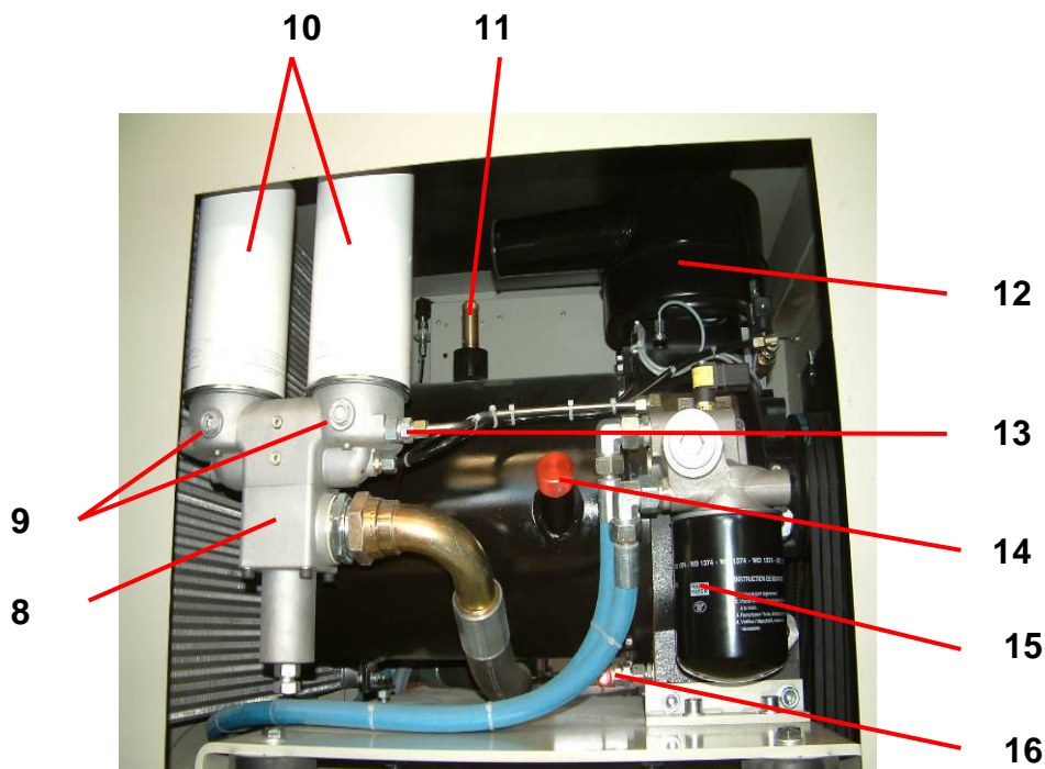
Изображение 2. Вид компрессора VEGA 56-75 сбоку.
