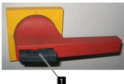
Рис. 6: Предохранение главного выключателя
