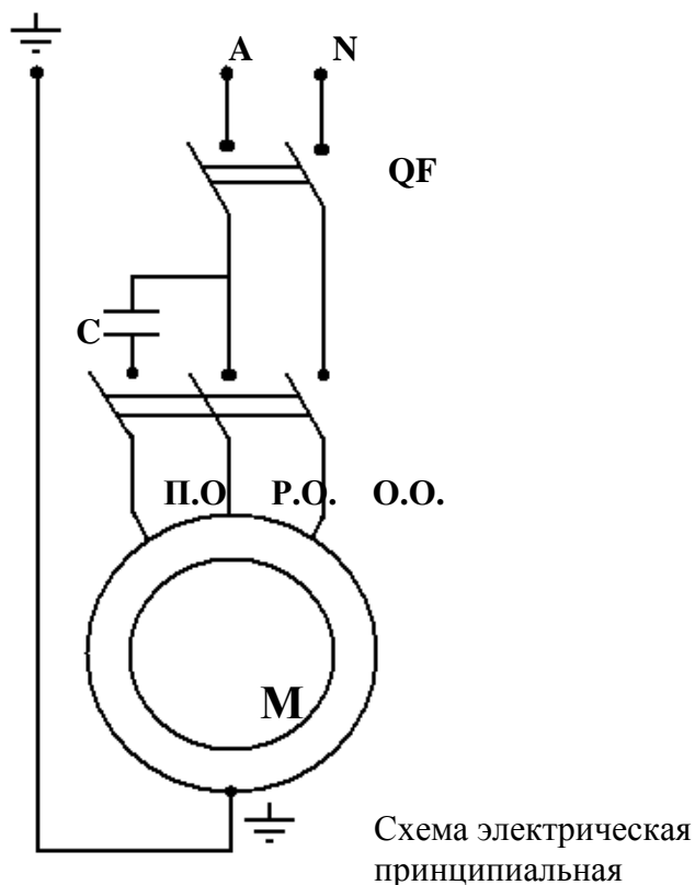
Схема подключения вибратора ИВ-98В, ИВ-99В
