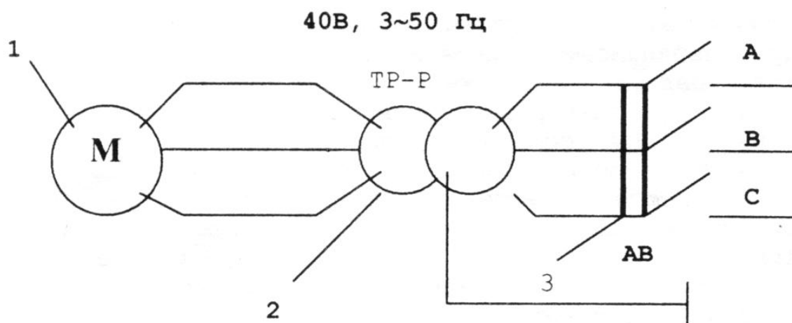
Схема подключения вибратора ИВ-98А, ИВ-99А
