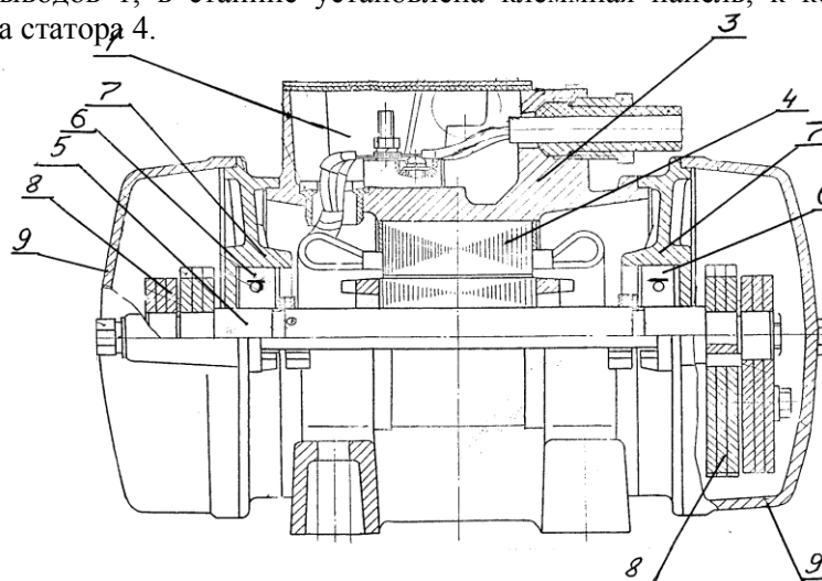
Рис. 2 Устройство вибраторов
