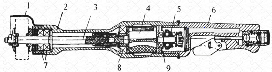
Рис. 1 Общий вид машины ИП-2009
