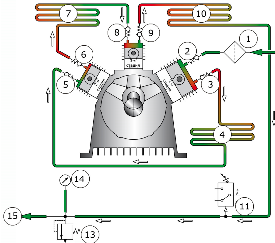
Рис. 14 Кругооборот давления
