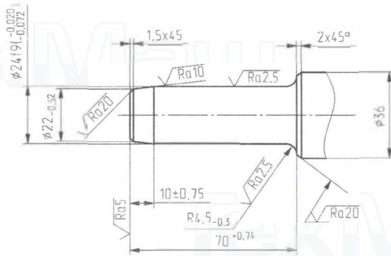
Рис. 4. Хвостовик инструмента для молотков МО-1Б, МО-2Б, МО-3Б, МО-4Б
