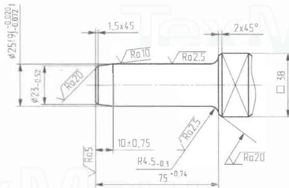
Рис. 6. Хвостовик инструмента для молотков МО-1БКУ, МО-2БКУ, МО-3БКУ, МО-4БКУ
