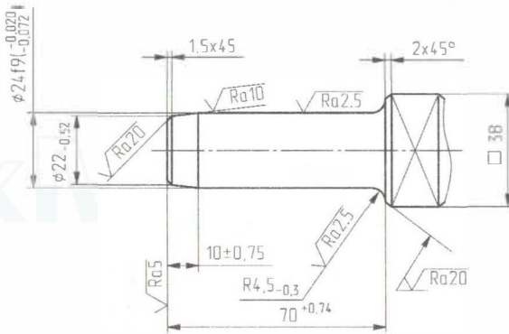
Рис. 5. Хвостовик инструмента для молотков МО-1БКС, МО-2БКС, МО-3БКС, МО-4БКС
