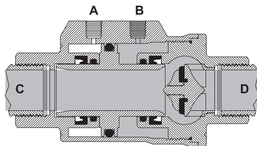
ОТКРЫТИЕ КЛАПАНА
