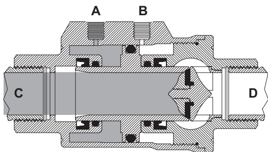
ЗАКРЫТИЕ КЛАПАНА
